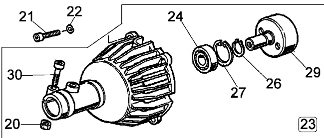
mod. 8220
