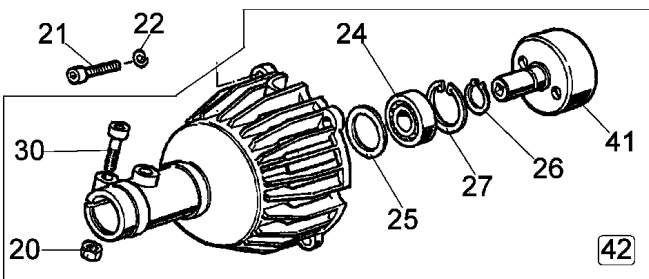
mod. 8200 Trimmer
